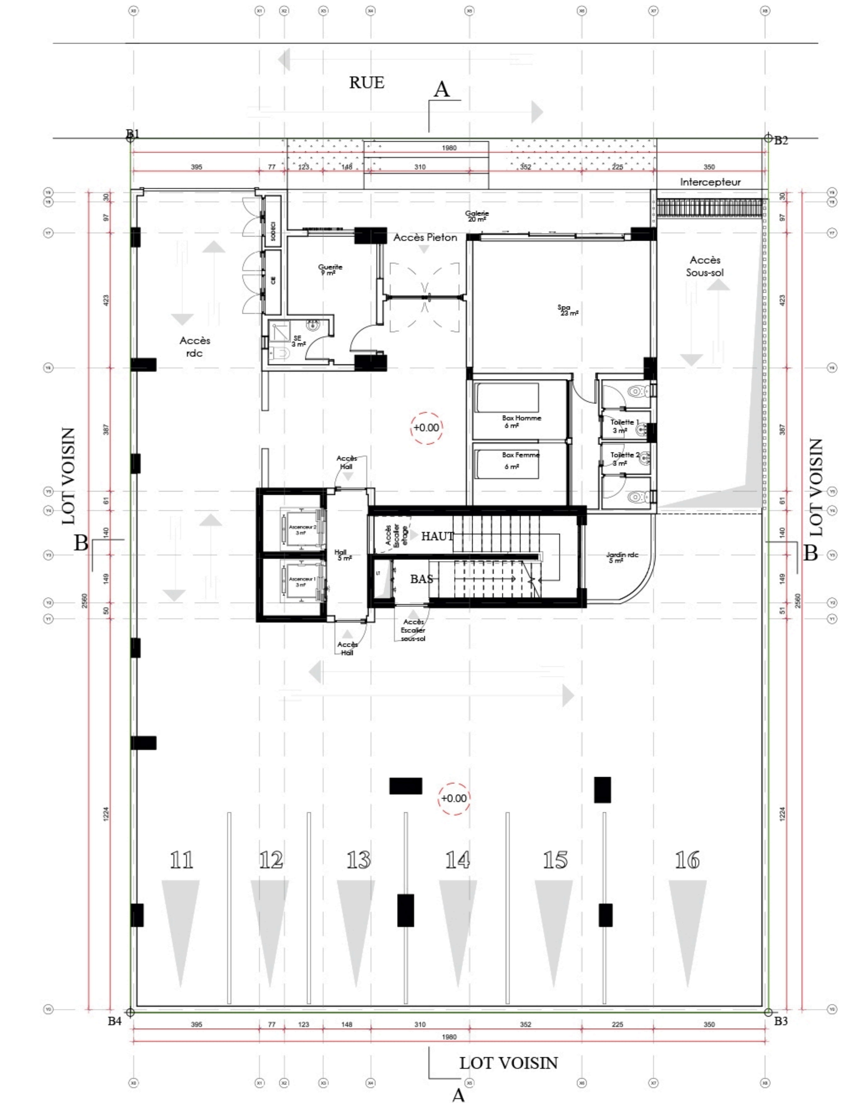
VUE EN PLAN RDC
