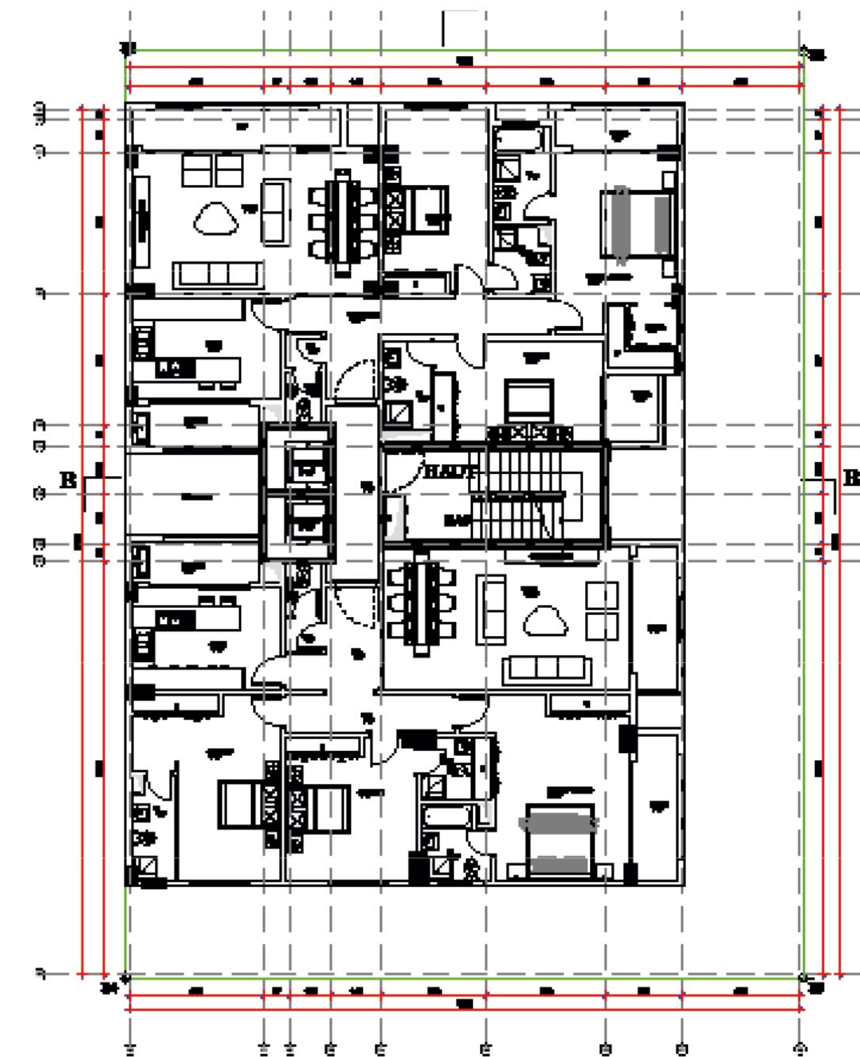
PLAN ETAGES COURANTS (ÉTAGE 1-6)
