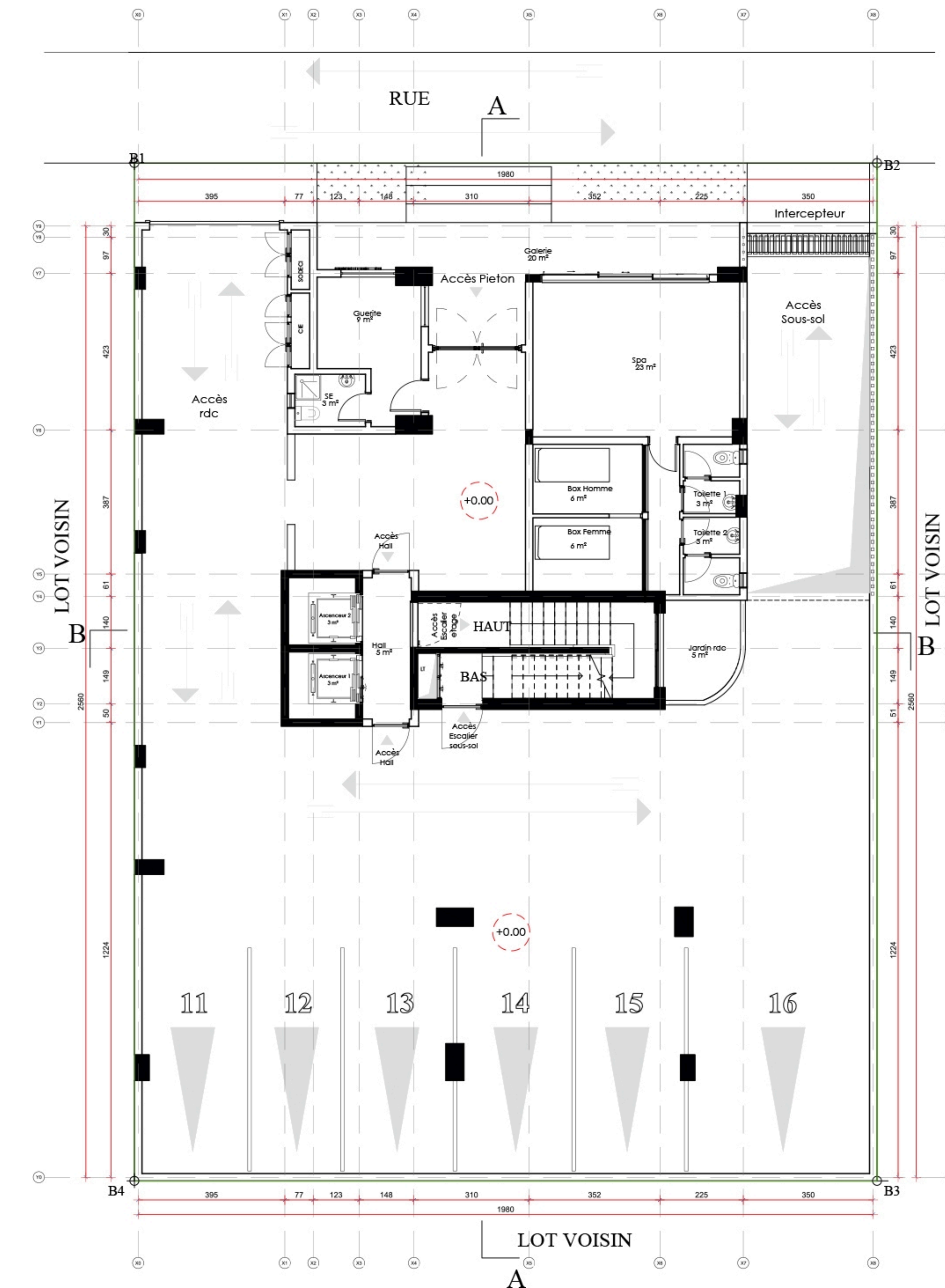
VUE EN PLAN RDC
