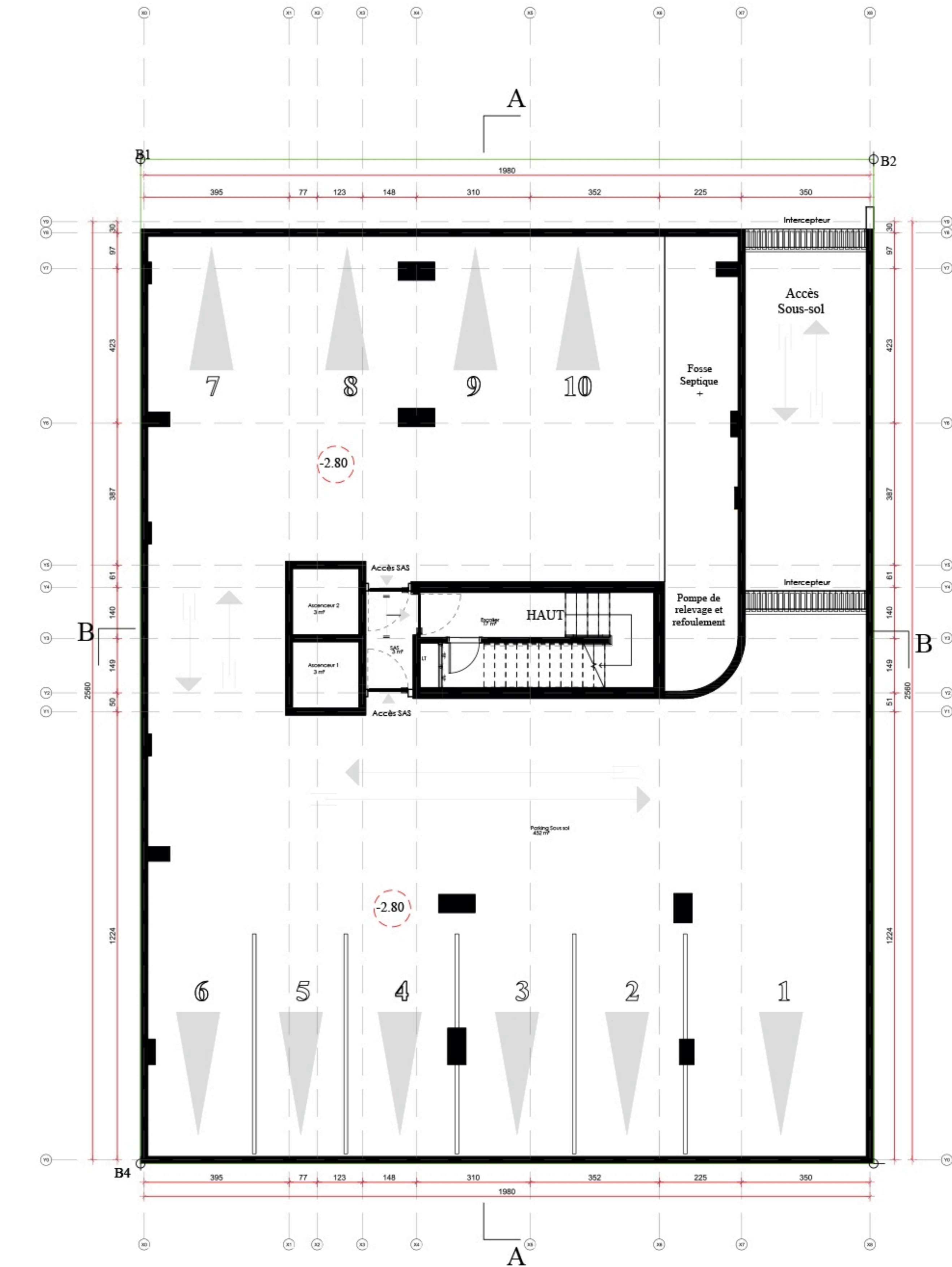
VUE EN PLAN SOUS-SOL
