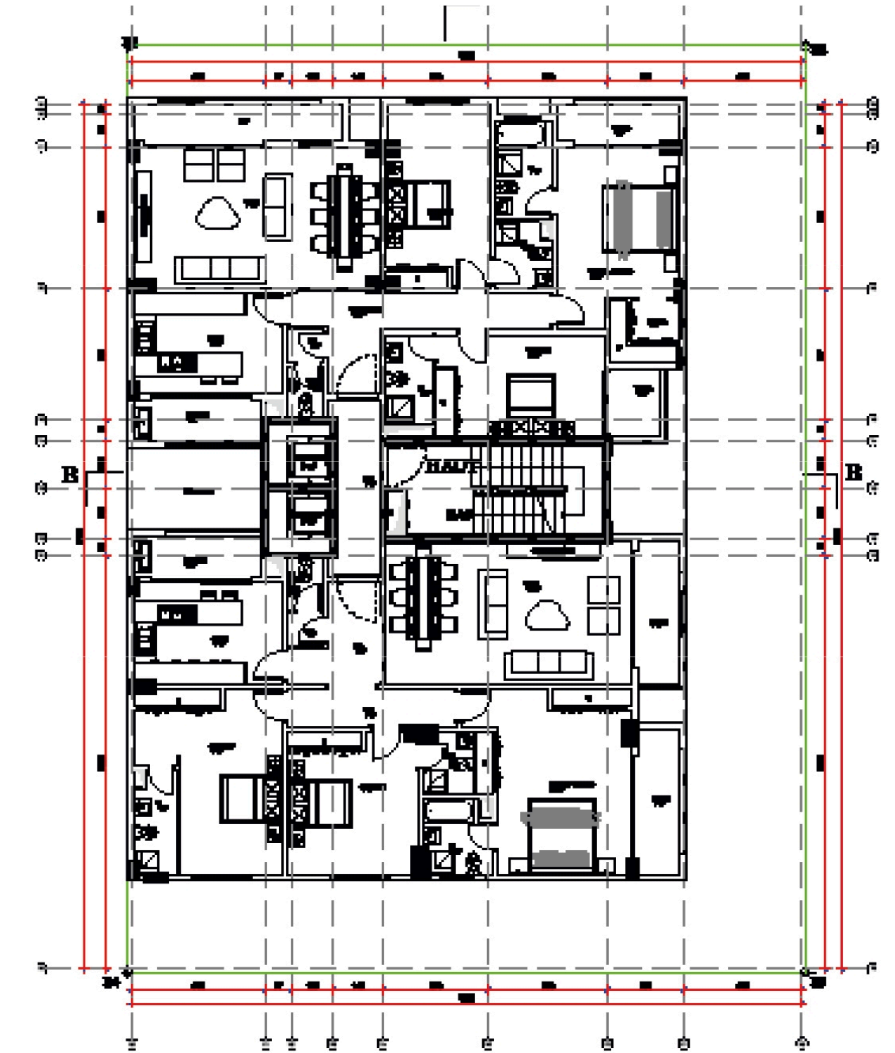
PLAN ETAGES COURANTS (ÉTAGE 1-6)
