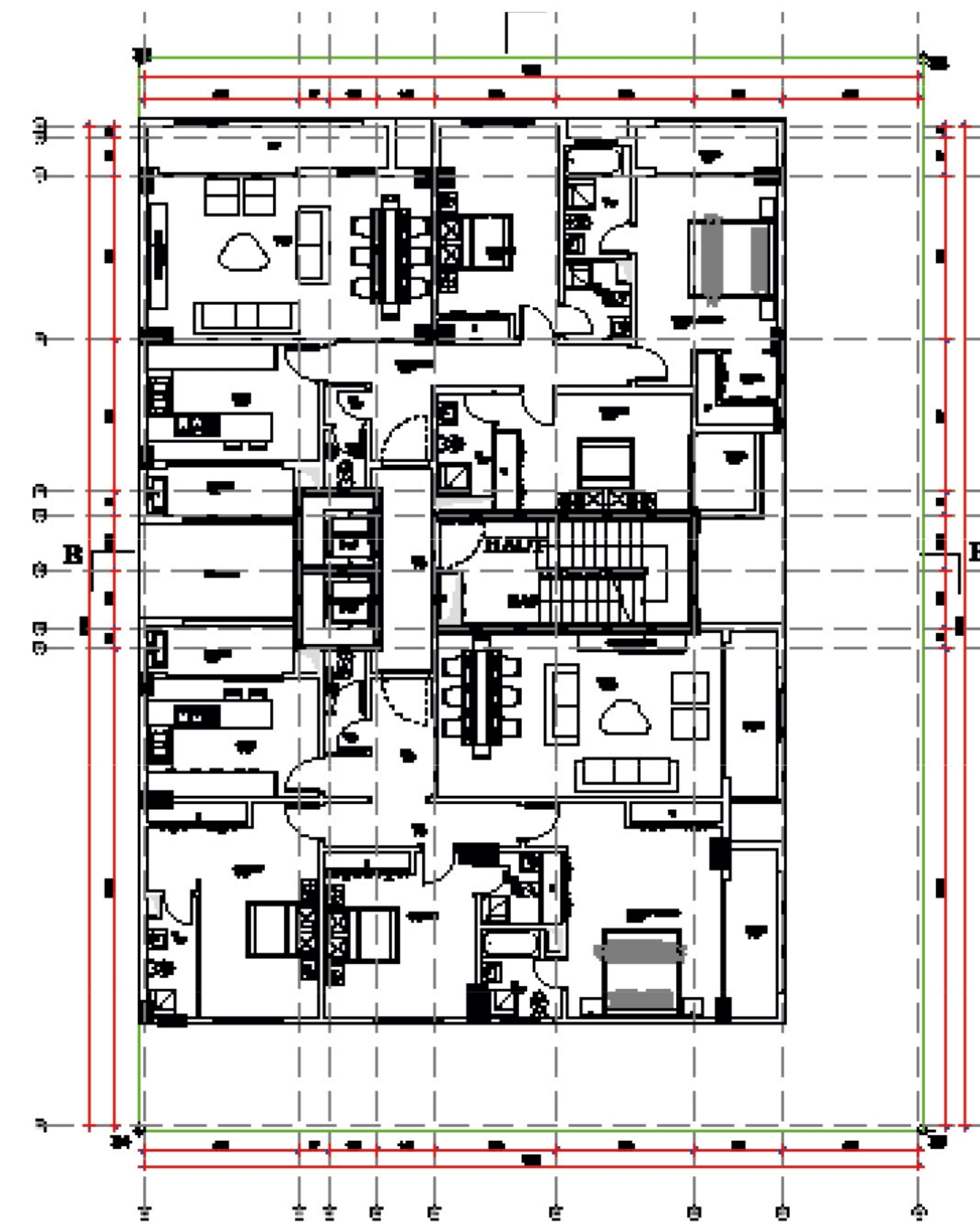
PLAN ETAGES COURANTS (ÉTAGE 1-6)
